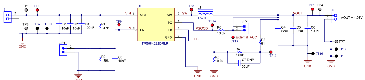
图 8-1. Schematic
