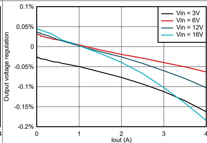
图 8-5. TPS564247 负载调整率与负载间的关系
