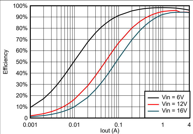
图 6-18. TPS564247 在 5V OUT 且使用 1.8 \mu H 电感器时的效率
