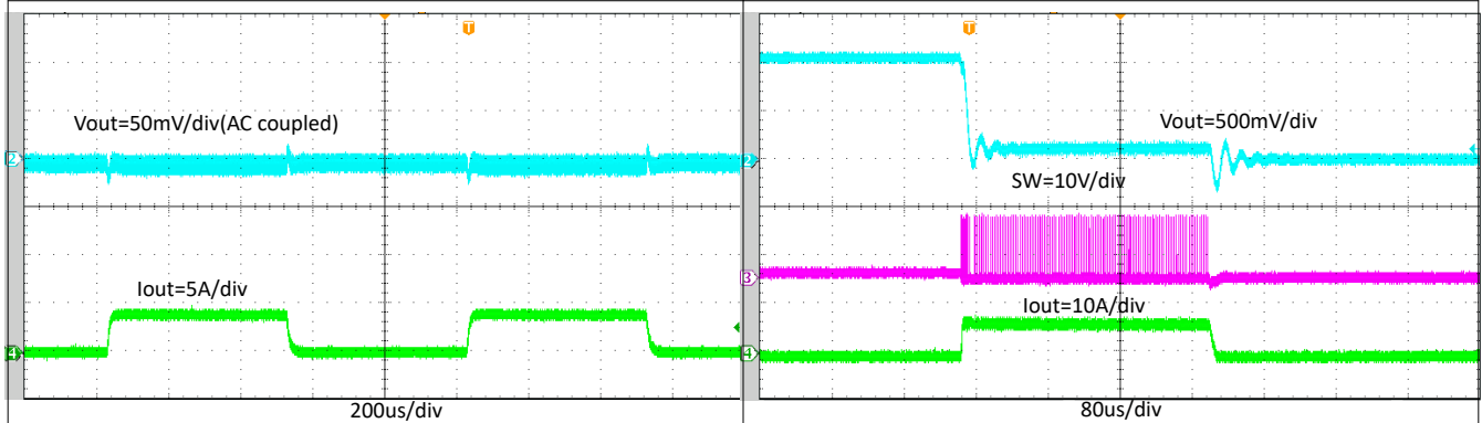
图 8-18. TPS564247 瞬态响应, 0.1A 至 4A, 负载阶跃为 2.5A/\mu s
