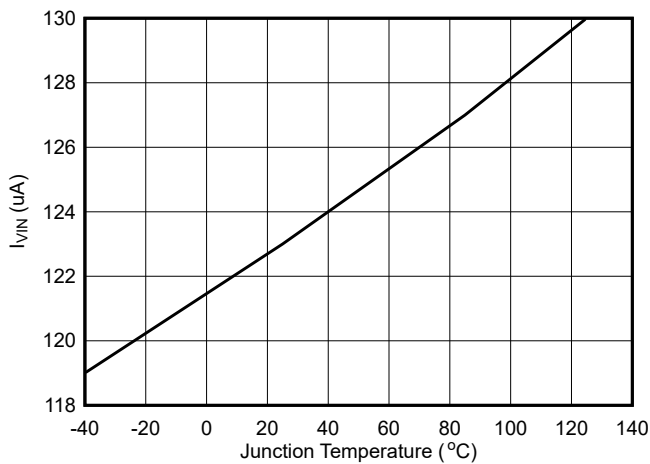
图 6-1. TPS564242 静态电流
