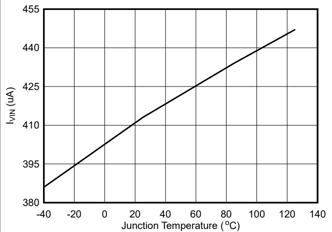
图 6-2. TPS564247 静态电流
