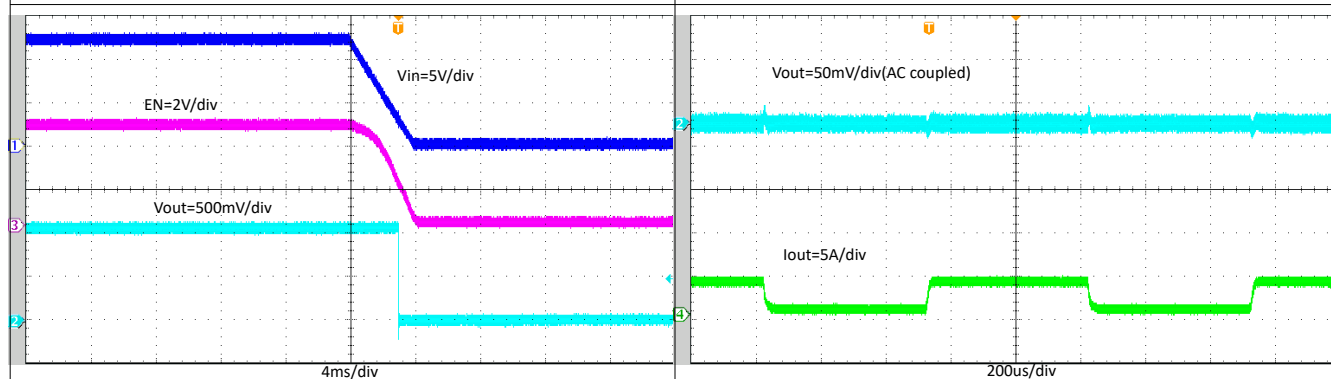
图 8-14. 在 V_{IN} 下降时启动, I_{OUT} = 4A
