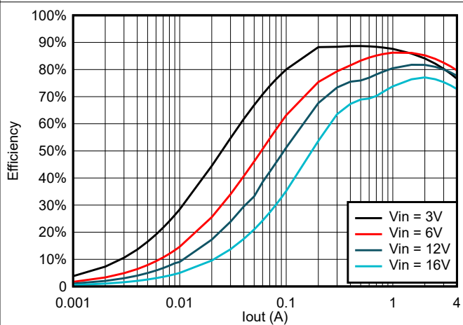
图 6-12. TPS564247 在 0.6V_{OUT} 且使用 0.82 \mu H 电感器时的效率
