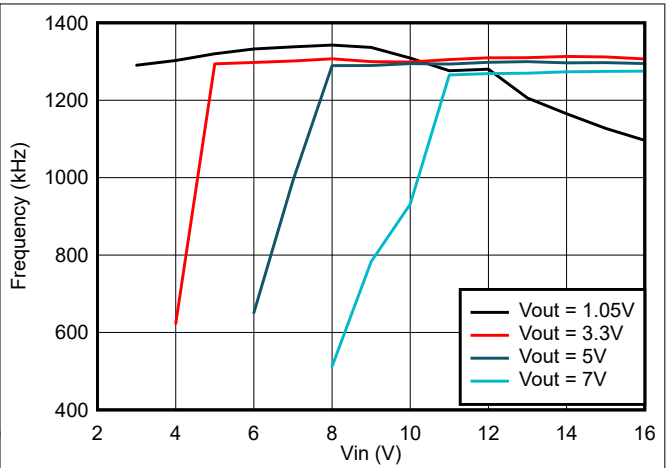
图 6-8. 4A 负载下频率与输入电压间的关系
