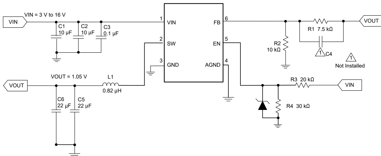
图 8-1. 原理图
