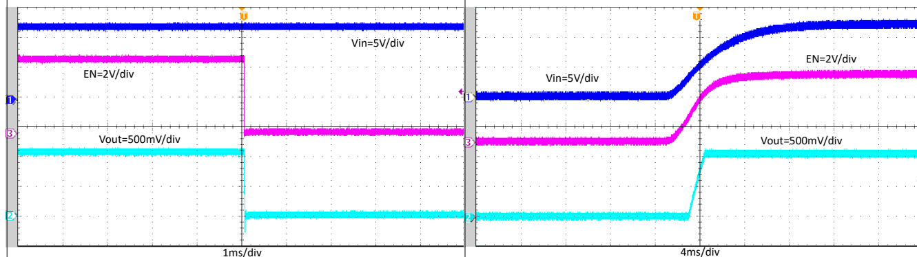
图 8-12. 通过 EN 关断, I_{OUT} = 4A
