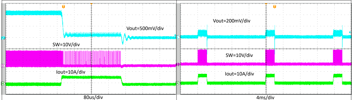
图 8-20. TPS564247 正常运行至输出硬短路
