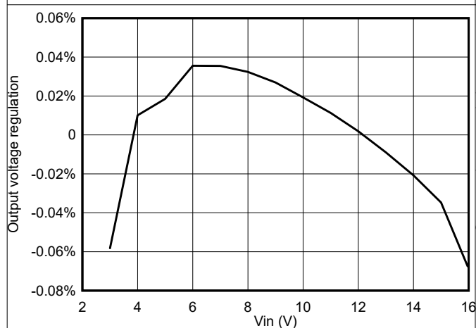
图 8-6. TPS564242 线性调整率与 V_{IN} 间的关系 (4A 负载)
