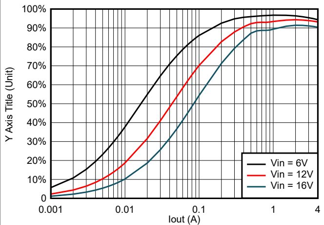
图 6-16. TPS564247 在 3.3V OUT 且使用 1.5 \mu H 电感器时的效率
