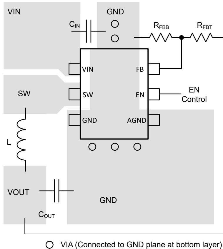
图 10-1. 建议的布局
