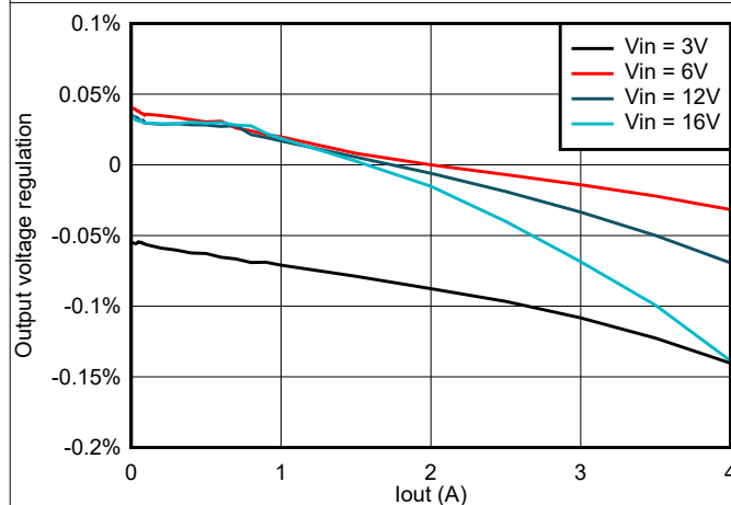
图 8-4. TPS564242 负载调整率与负载间的关系
