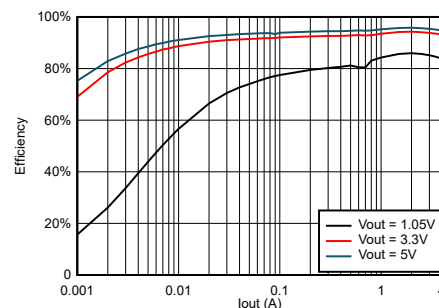
TPS564242 在 V_{IN} = 12V 时的效率
