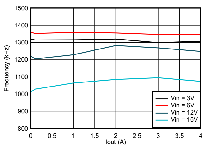
图 8-3. TPS564247 频率与负载间的关系
