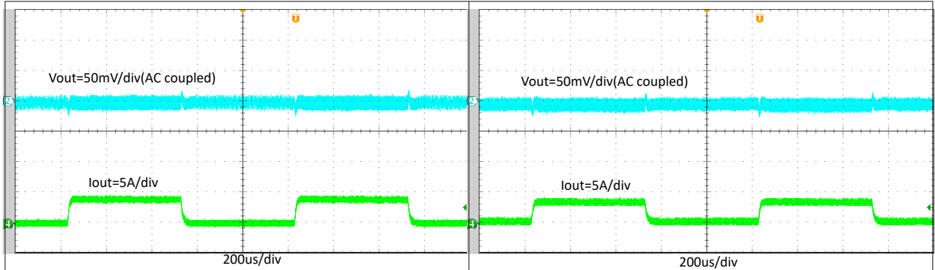
图 8-16. TPS564242 瞬态响应, 0.1A 至 4A, 负载阶跃为 2.5A/\mu s
