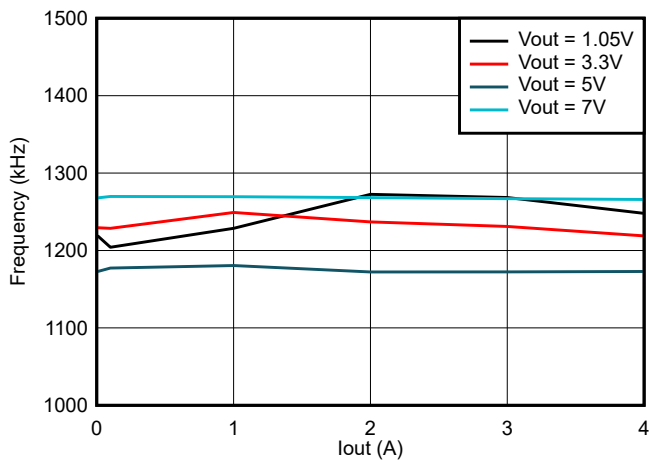
图 6-9. TPS564247 频率与负载间的关系
