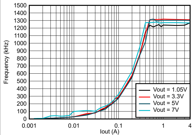
图 6-10. TPS564242 频率与负载间的关系
