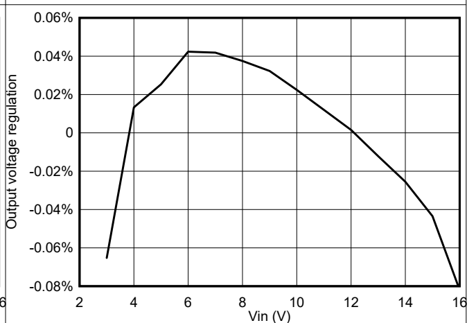
图 8-7. TPS564247 线性调整率与 V_{IN} 间的关系 (4A 负载)
