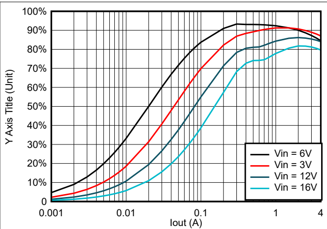
图 6-14. TPS564247 在 1.05V OUT 且使用 0.82 \mu H 电感器时的效率
