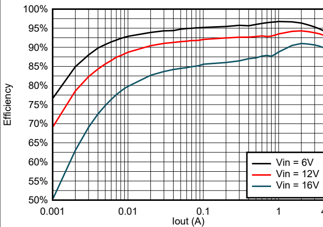
图 6-15. TPS564242 在 3.3V OUT 且使用 1.5 \mu H 电感器时的效率
