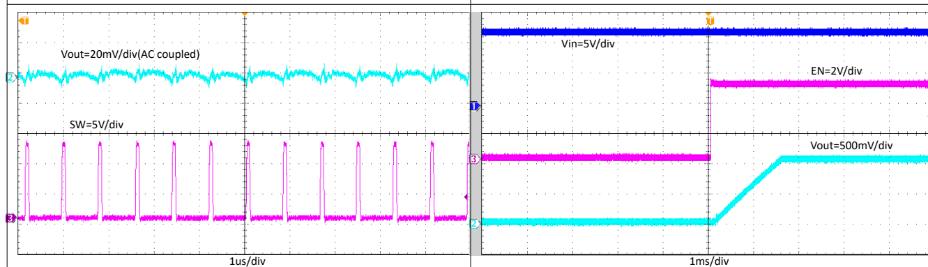
图 8-10. 输出电压纹波 (4A 负载)
