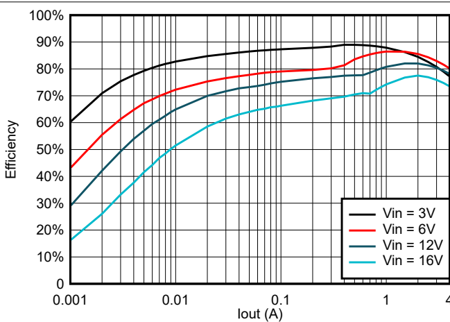
图 6-11. TPS564242 在 0.6V_{OUT} 且使用 0.82 \mu H 电感器时的效率
