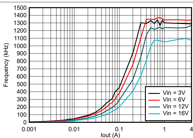
图 8-2. TPS564242 频率与负载间的关系
