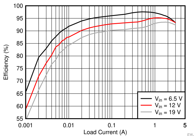
图 18. Efficiency
