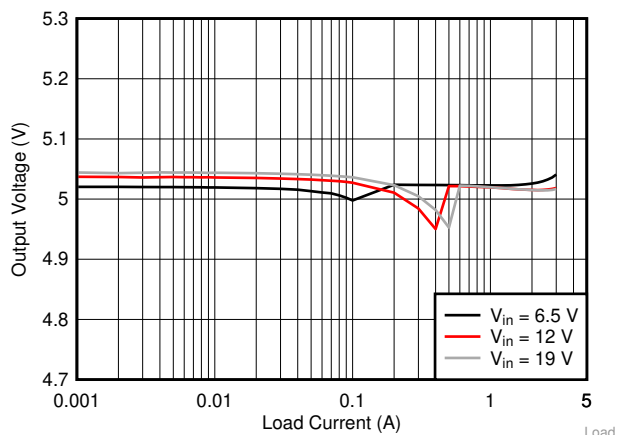
图 19. Load Regulation
