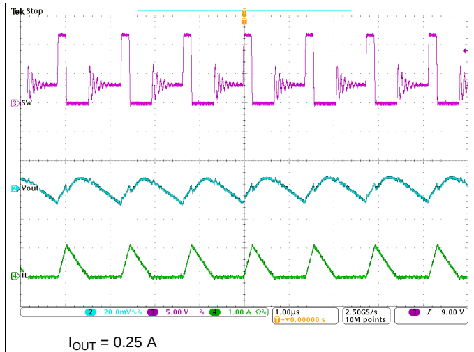
图 27. Output Voltage Ripple
