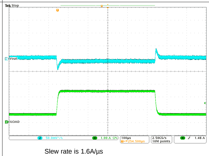
图 29. Transient Response, 0.6 to 2.4A
