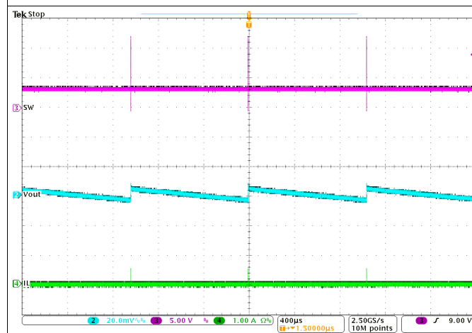
图 24. Output Voltage Ripple
