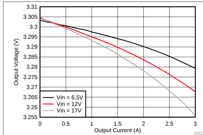
图 20. Load Regulation
