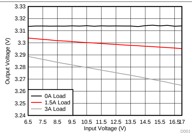
图 21. Line Regulation
