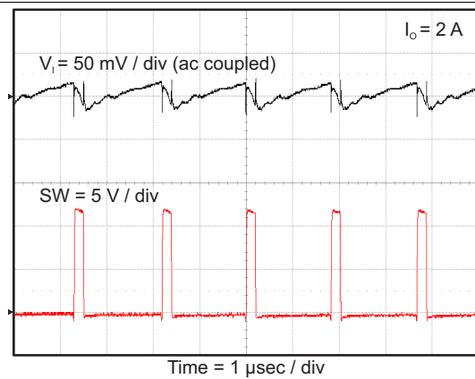
图 23. TPS562219A Input Voltage Ripple
