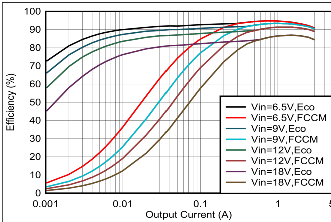
图 8-2. Efficiency
