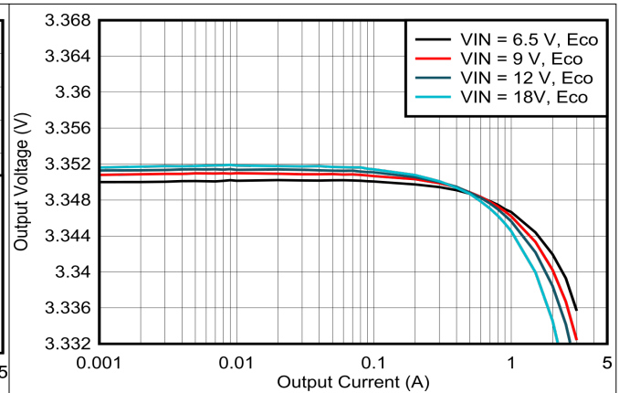
图 8-3. Load Regulation
