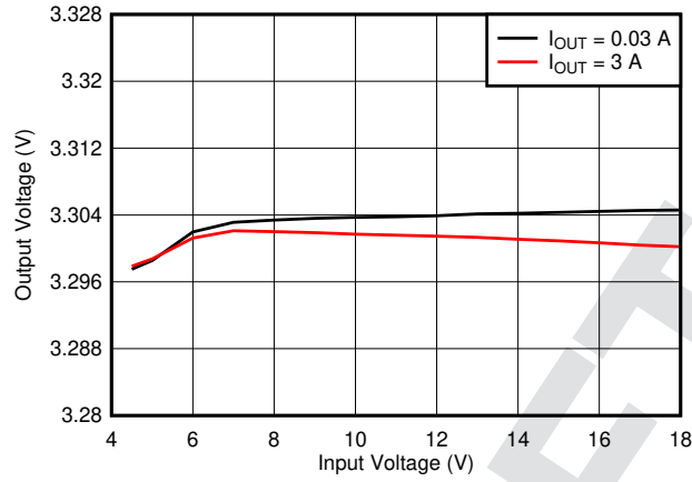
图 8-4. 线路调节
