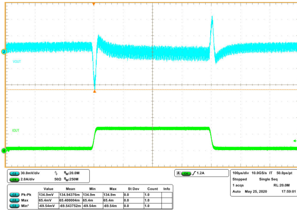
图 8-14. 瞬态响应为 0.3 至 2.7A，压摆率 0.25A/\mu s
