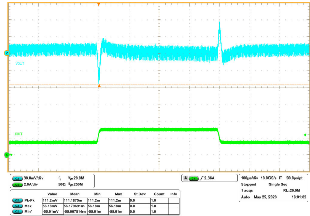
图 8-15. 瞬态响应为 1.5 至 3A，压摆率 0.25A/\mu s
