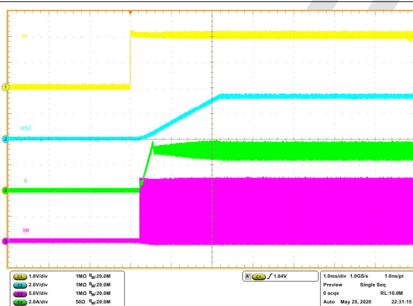
图 8-18. 相对于 EN 的启用
