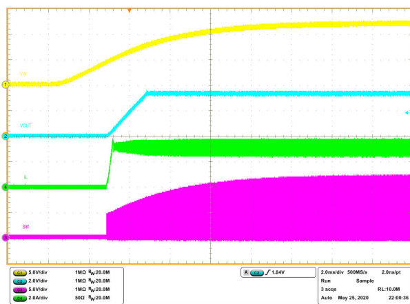
图 8-16. 相对于 VIN 的启动
