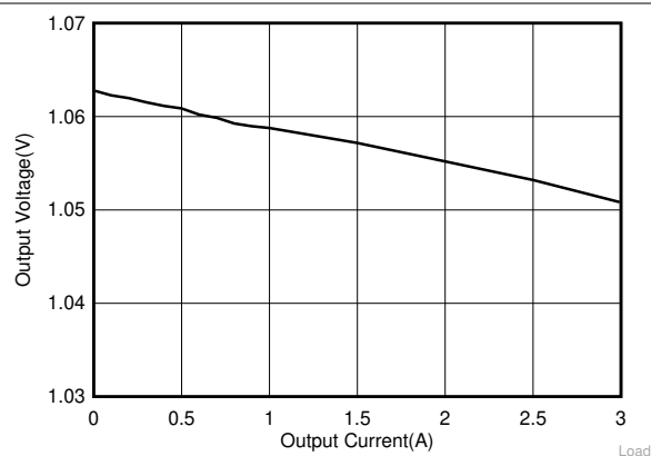
图 9-2. 不同负载的负载调节
