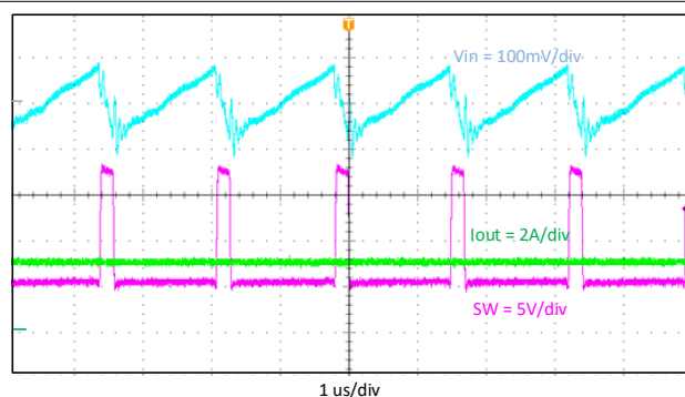
图 9-4. 输入电压纹波 I_{out} = 3A
