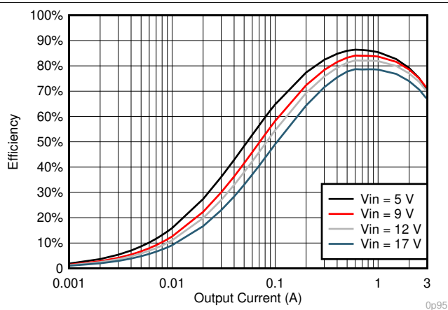
图 7-9. V_{OUT} = 0.95V 效率, L = 1.5\mu H
