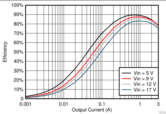
图 7-11. V_{OUT} = 1.5V 效率, L = 2.2\mu H
