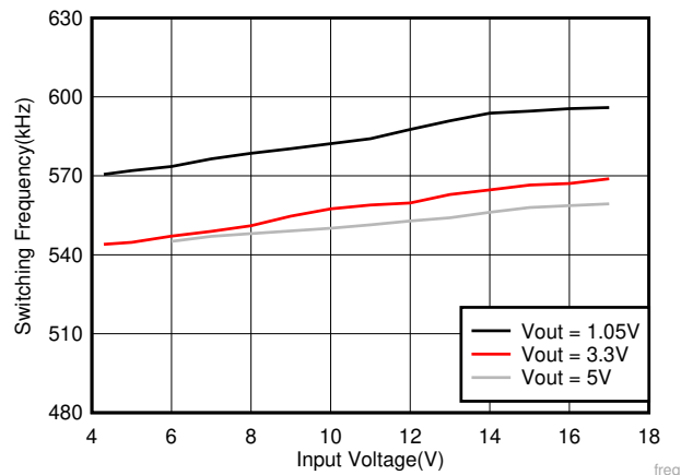
图 7-7. 开关频率与输入电压间的关系
