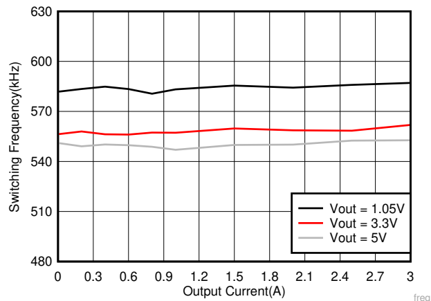
图 7-8. 开关频率与输出电流间的关系
