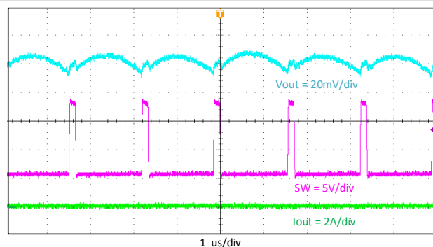
图 9-6. 输出电压纹波, I_{out} = 10mA
