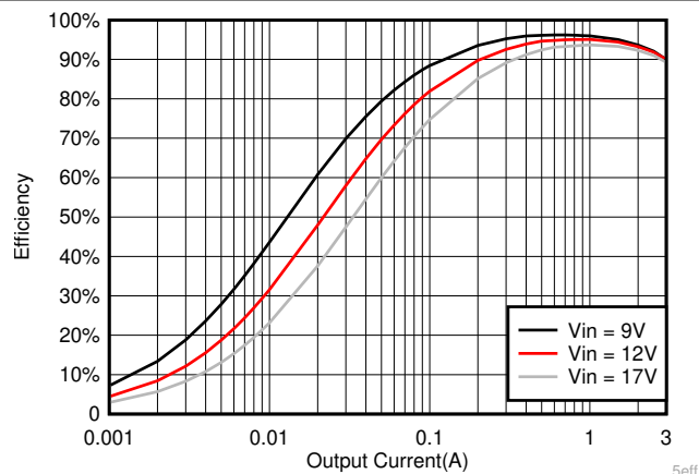
图 7-14. V_{OUT} = 5V 效率, L = 4.7\mu H
