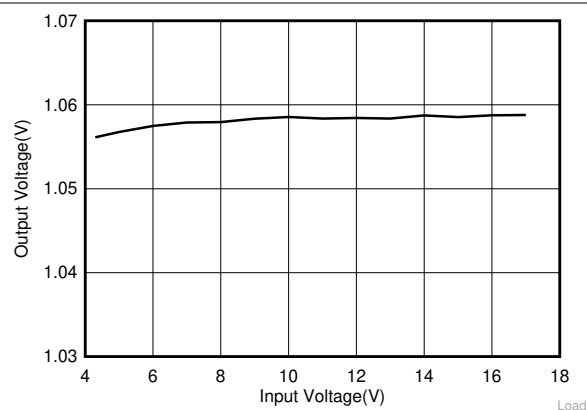
图 9-3. 不同输入电压的负载调节
