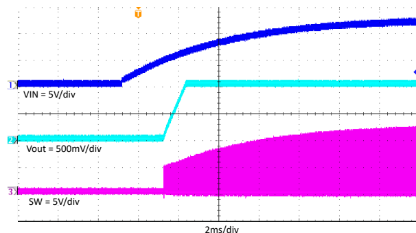
图 7-18. TPS563206 在负载电流为 3A 时上电
