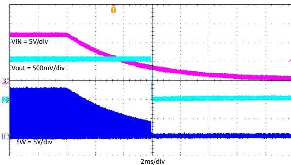
图 7-17. TPS563203 在负载电流为 3A 时断电
