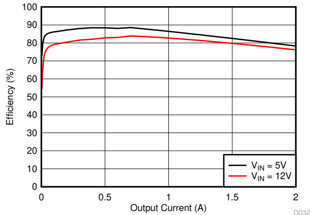
图 8-2. Tps562200 Efficiency
