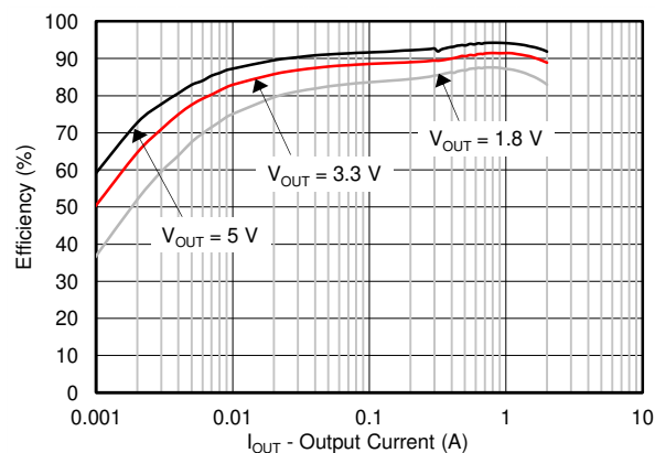
TPS562200 效率
