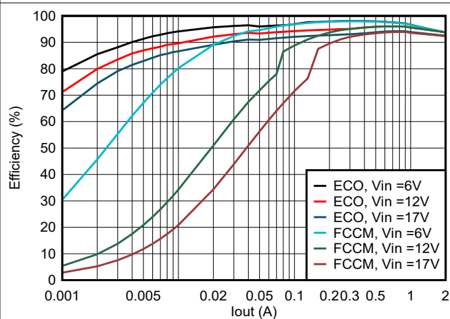
图 5-12. TPS56224x 在 5Vout 且使用 3.3uH 电感器时的效率
