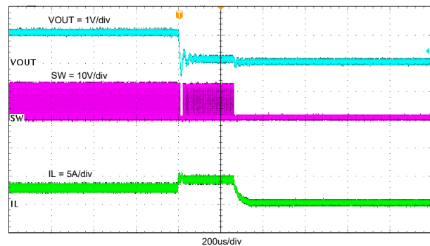
图 7-17. TPS562246 正常运行至输出硬短路
