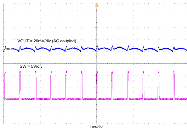
图 7-3. TPS562246 输出电压纹波 (0.01A 负载)
