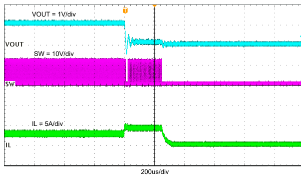
图 7-16. TPS562243 正常运行至输出硬短路
