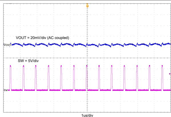
图 7-4. TPS562243 输出电压纹波 (2A 负载)
