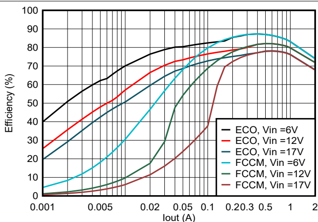
图 5-9. TPS56224x 在 0.6Vout 且使用 1uH 电感器时的效率
