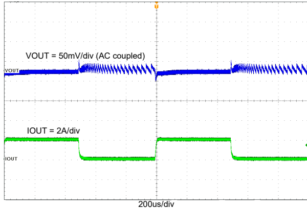
图 7-14. TPS562243 电流为 0A 至 2A 时的负载瞬态
