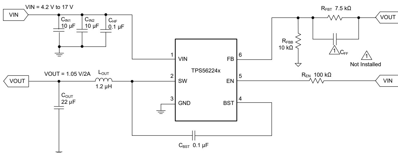
图 7-1. TPS56224x 1.05V/2A 参考设计
