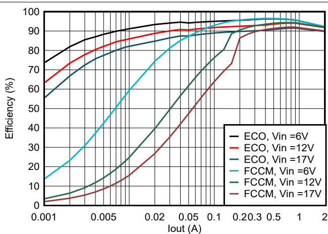
图 5-11. TPS56224x 在 3.3Vout 且使用 2.2uH 电感器时的效率
