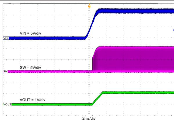
图 7-10. TPS562243 在负载电流为 2A 时上电
