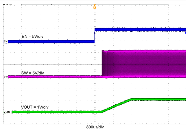
图 7-6. TPS562243 在负载电流为 2A 时使能开
