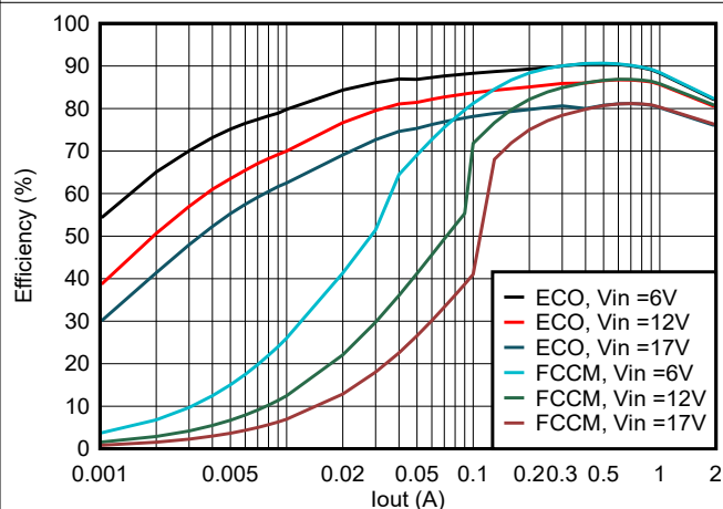
图 5-10. TPS56224x 在 1.05Vout 且使用 1.2uH 电感器时的效率
