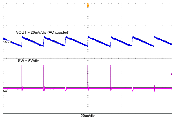
图 7-2. TPS562243 输出电压纹波 (0.01A 负载)
