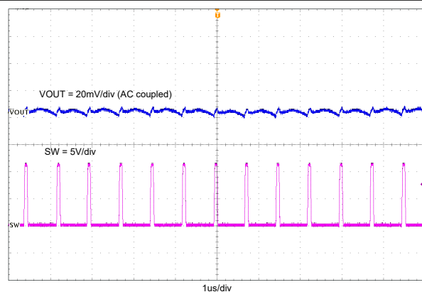
图 7-5. TPS562246 输出电压纹波 (2A 负载)
