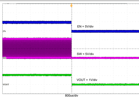
图 7-7. TPS562243 在负载电流为 2A 时使能关
