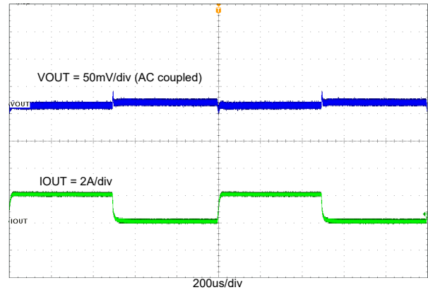
图 7-15. TPS562246 电流为 0A 至 2A 时的负载瞬态
