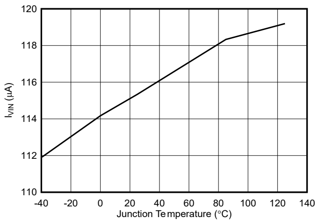
图 5-1. TPS562243 静态电流
