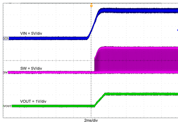
图 7-12. TPS562246 在负载电流为 2A 时上电
