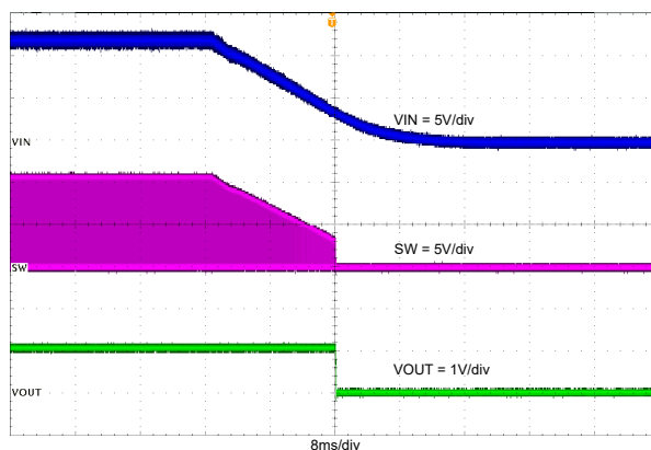
图 7-13. TPS562246 在负载电流为 2A 时断电
