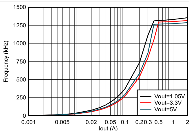
图 5-8. TPS562243 频率与负载间的关系
