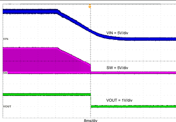
图 7-11. TPS562243 在负载电流为 2A 时断电
