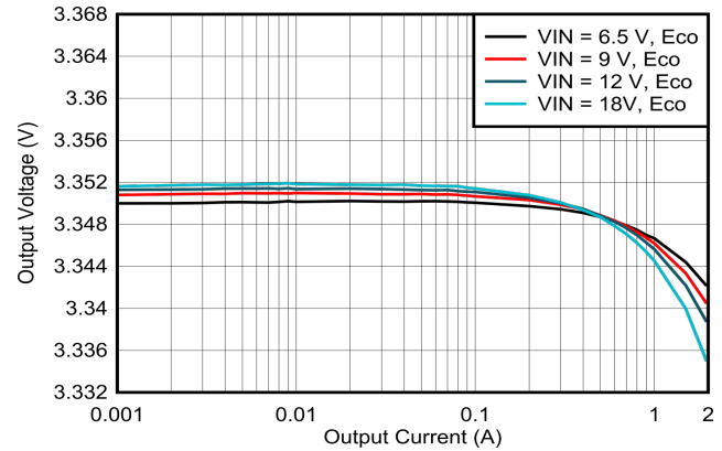
图 8-3. Load Regulation
