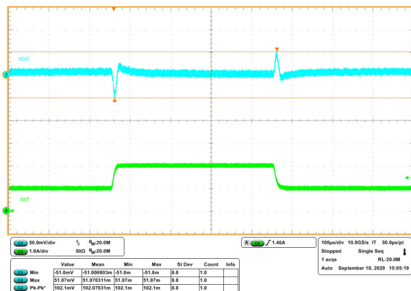
图 8-15. 瞬态响应 1 至 2A，压摆率 0.25\text{A}/\mu\text{s}
