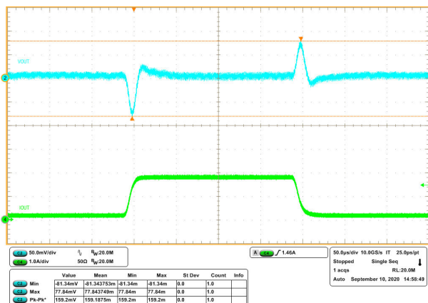
图 8-14. 瞬态响应 0.2 至 1.8A，压摆率 0.25\text{A}/\mu\text{s} (FCCM)
