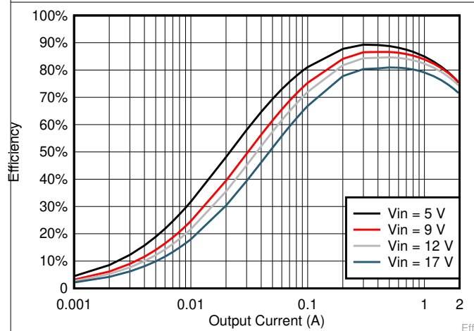
图 6-9. V_{OUT} = 0.95V 效率, L = 2.2\mu H
