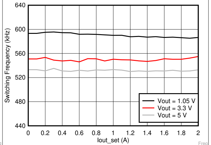
图 6-8. 开关频率与输出电流间的关系
