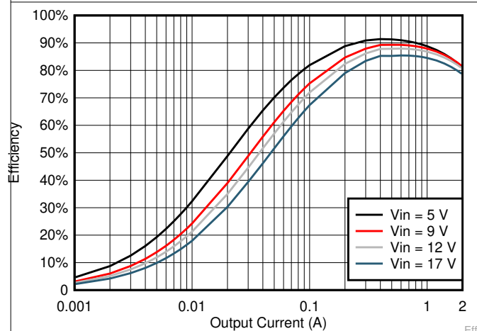
图 6-11. V_{OUT} = 1.5V 效率, L = 2.2\mu H
