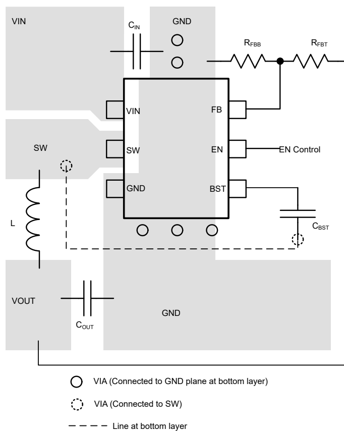
图 7-22. TPS562203 布局
