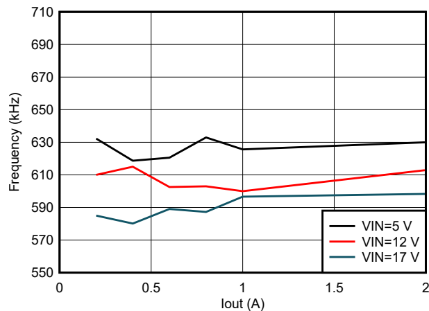
图 7-3. TPS562206 频率与负载间的关系
