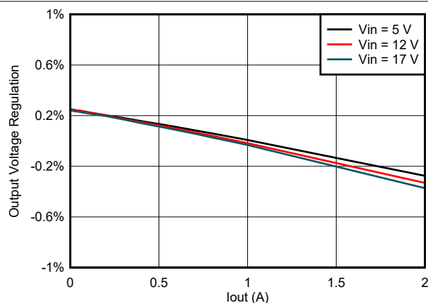
图 7-5. TPS562206 负载调整率与负载间的关系
