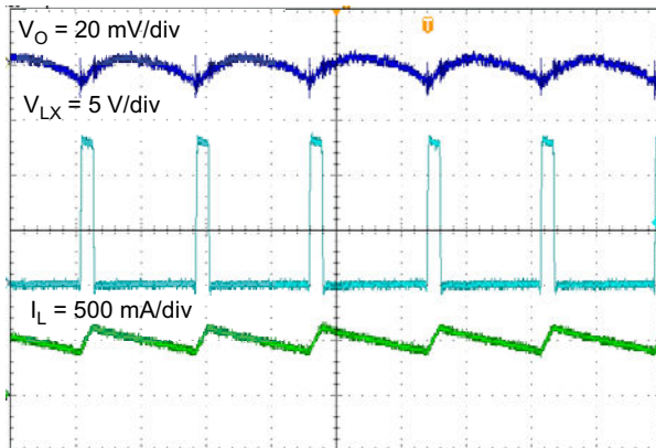
图 7-9. TPS562201 Output Voltage Ripple, I_{OUT} = 2 \text{ A}
