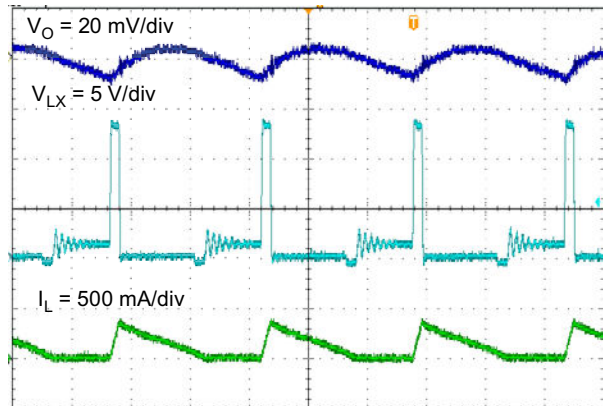
图 7-8. TPS562201 Output Voltage Ripple, I_{OUT} = 0.25 \text{ A}
