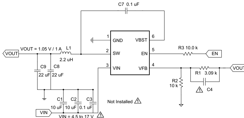
图 8-1. TPS561201 和 TPS561208 1.05-V/1-A 参考设计
