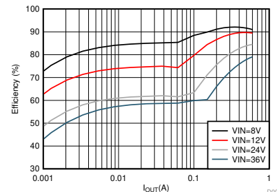
效率与输出电流间的关系 V_{\text{OUT}} = 5\text{V} , 2100kHz, PFM
