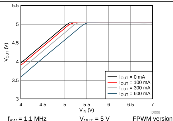
图 8. Dropout
