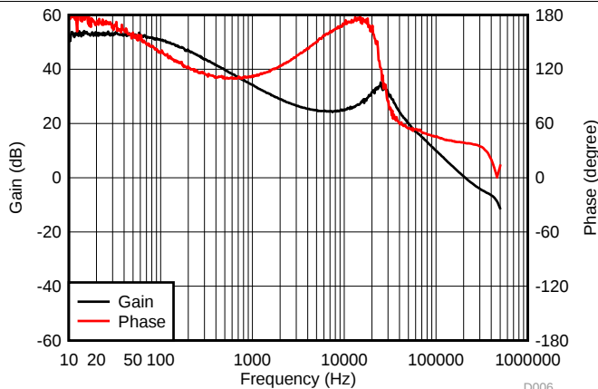
图 12. Loop Response, I_{OUT} = 0.25\text{ A}
