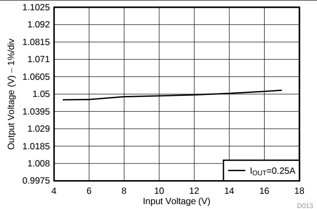
图 11. Line Regulation
