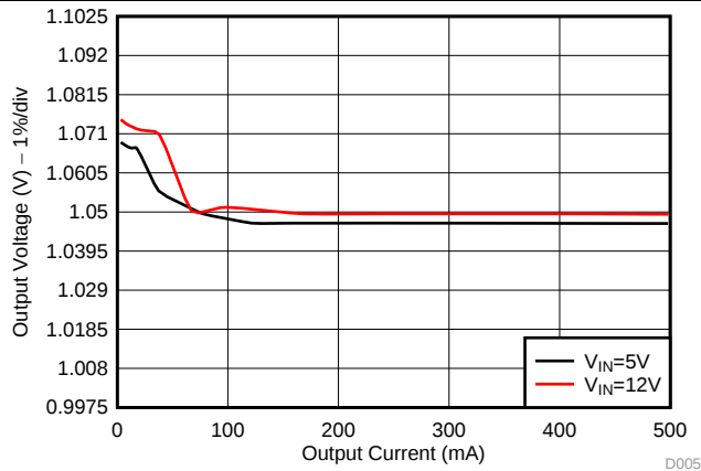
图 10. Load Regulation
