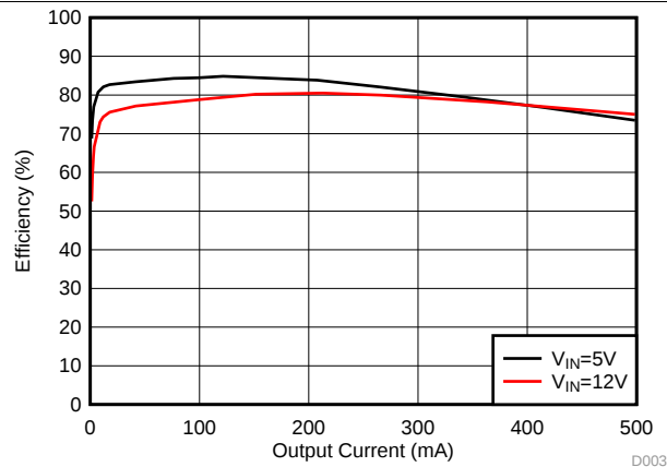
图 8. Efficiency
