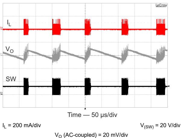
图 8-7. Pulse Skipping
