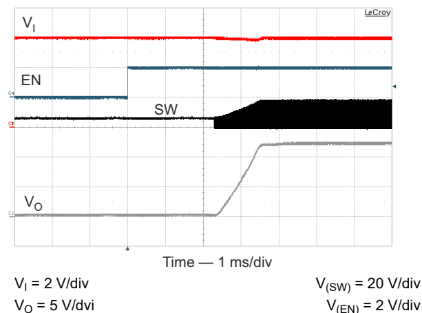
图 8-15. Output Voltage Soft Start
