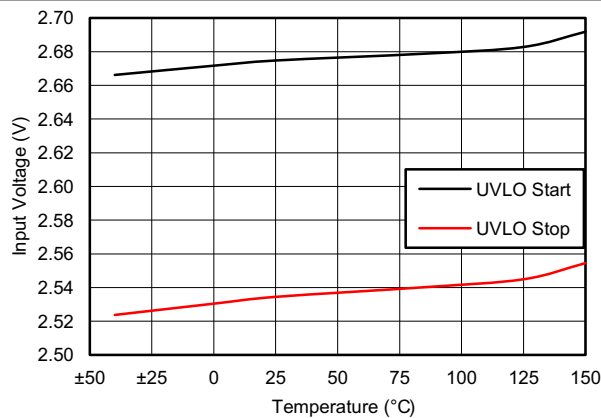
图 6-11. Input Voltage UVLO vs Temperature
