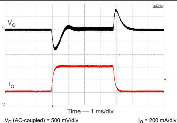
图 8-4. Load Transient Response
