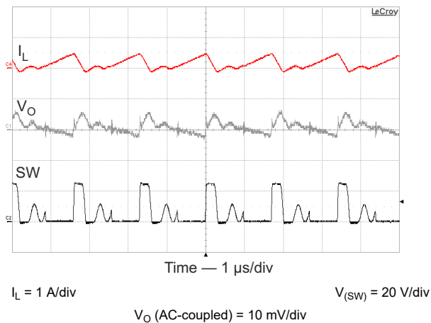
图 8-6. DCM PWM Operation
