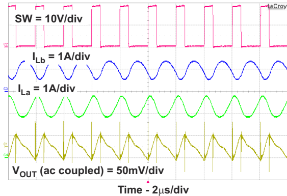
图 9-14. CCM PWM Operation
