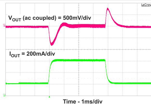
图 9-4. Load Transient Response
