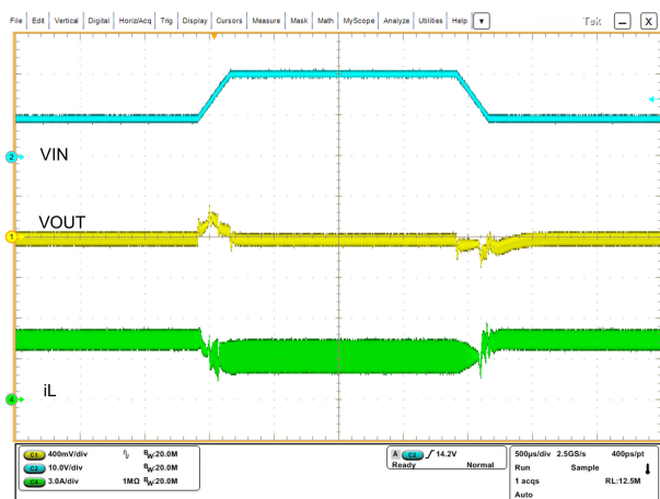
图 8-10. V_{IN} = 9V 至 20V 、 V_{OUT} = 12V 、 I_O = 3A 、 200\mu s 转换率时的线路瞬态波形，FPWM
