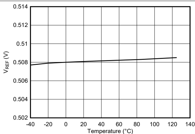
图 5-13. 基准电压与温度间的关系 ( V_{REF} = 0.508V )
