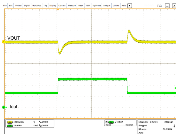
图 8-11. V_{IN} = 12V 、 V_{OUT} = 5V 、 I_O = 2.5A 至 5A 、 20\mu s 转换率时的负载瞬态波形, FPWM
