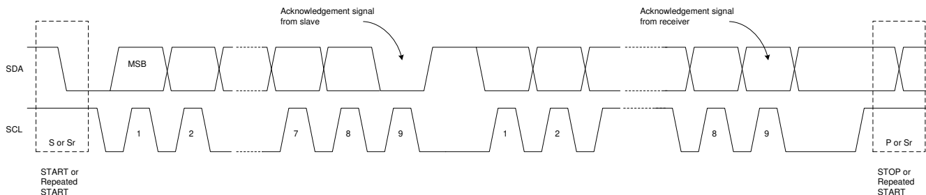
图 7-9. Byte Format
