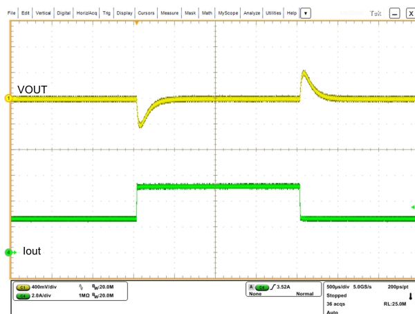
图 8-11. V_{IN} = 12V 、 V_{OUT} = 5V 、 I_O = 2.5A 至 5A 、 20\mu s 转换率时的负载瞬态波形 (FPWM 模式)
