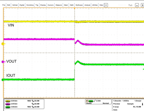
图 8-12. V_{IN} = 12V 、 V_{OUT} = 5V 、 R_{LOAD} = 1\Omega 、 R_{SNS} = 10m\Omega 时的 3A 输出电流限制波形，（FPWM 模式）
