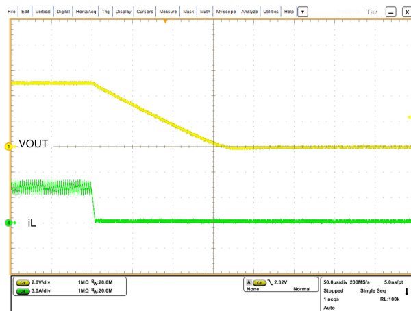
图 8-9. V_{IN} = 12V 、 V_{OUT} = 5V 、 R_{LOAD} = 1.2\Omega 时的关断波形 (FPWM 模式)
