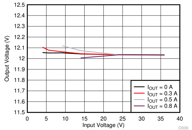
图 7-6. 12-V Output Regulation vs Input Voltage
