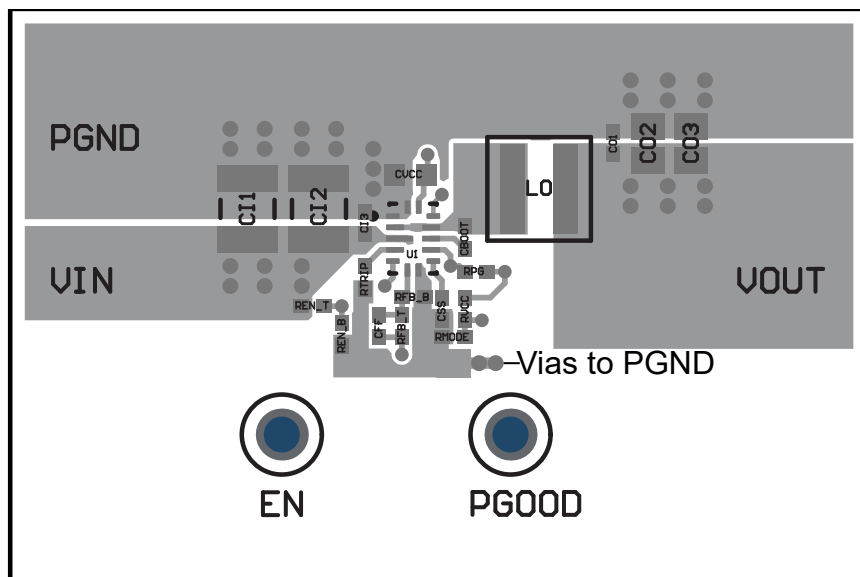
图 7-33. 顶层布局
