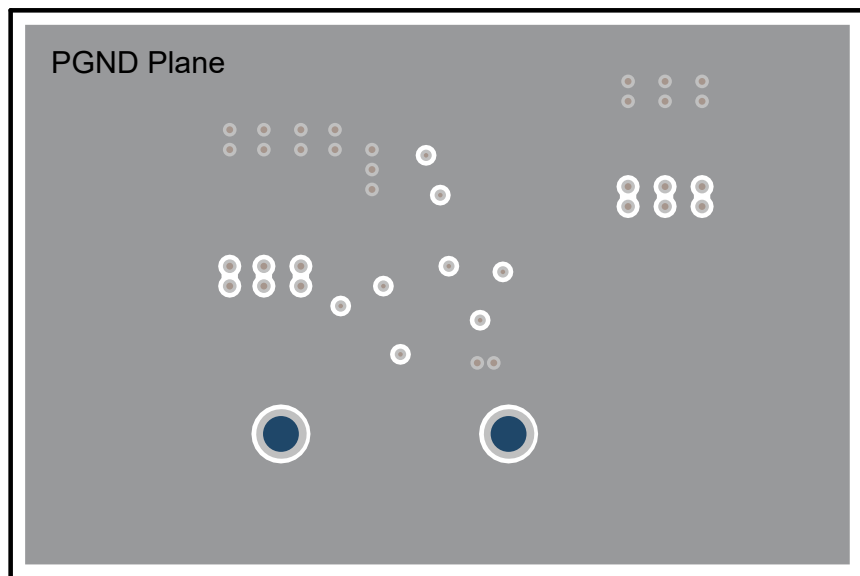
图 7-34. 信号层 1 布局
