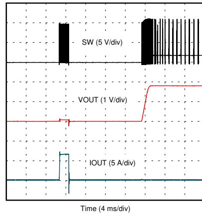
图 7-32. 过流退出断续模式
