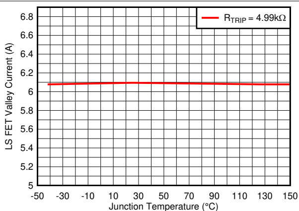
图 5-3. 过流限值
