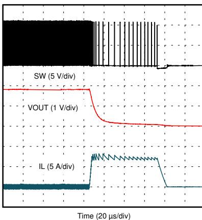
图 7-30. 短路响应
