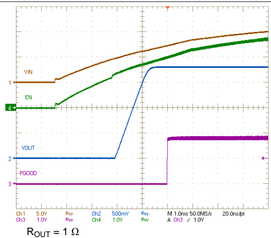
图 48. V_{IN} Start-up
