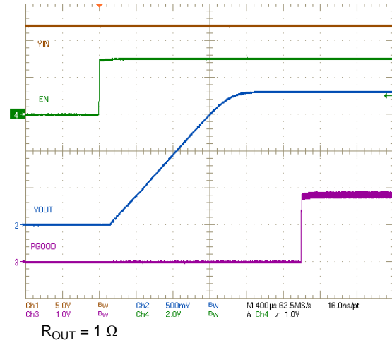
图 50. EN Start-up
