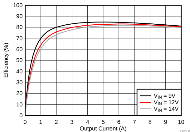
图 48. Efficiency
