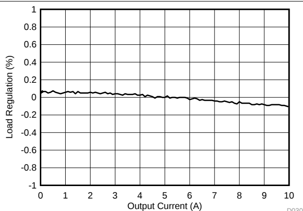
图 50. Load Regulation
