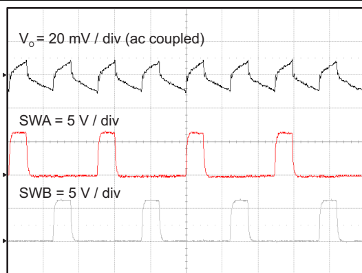
图 56. No Load Output Voltage Ripple
