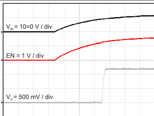
图 58. Start Up with VIN
