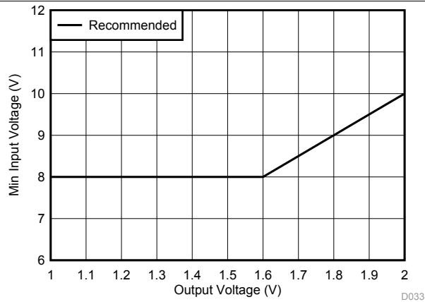
图 25. Min Input Voltage vs Output Voltage
