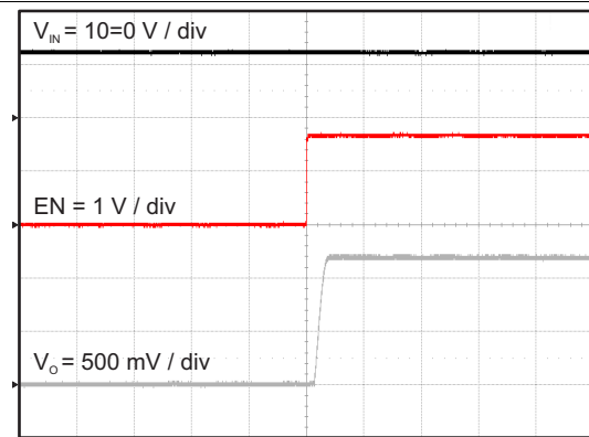
图 59. Start Up with EN
