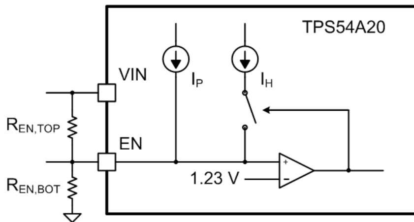
图 42. Adjustable VIN Undervoltage Lockout
