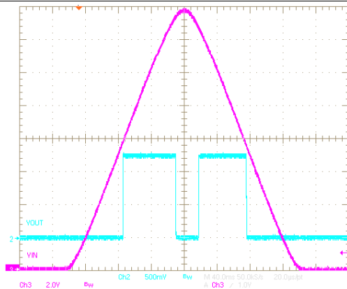
图 25. Min Input Voltage vs Output Voltage
