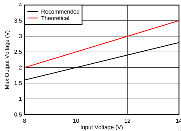
图 24. Max Output Voltage vs Input Voltage
