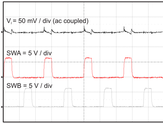
图 54. No Load Input Voltage Ripple
