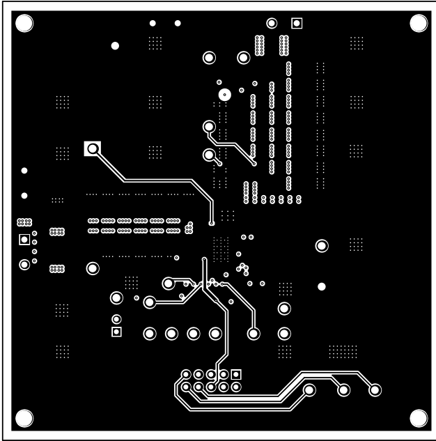
图 67. EVM Inner Layer 3
