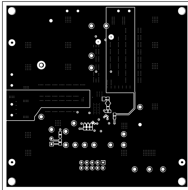
图 69. EVM Bottom Layer
