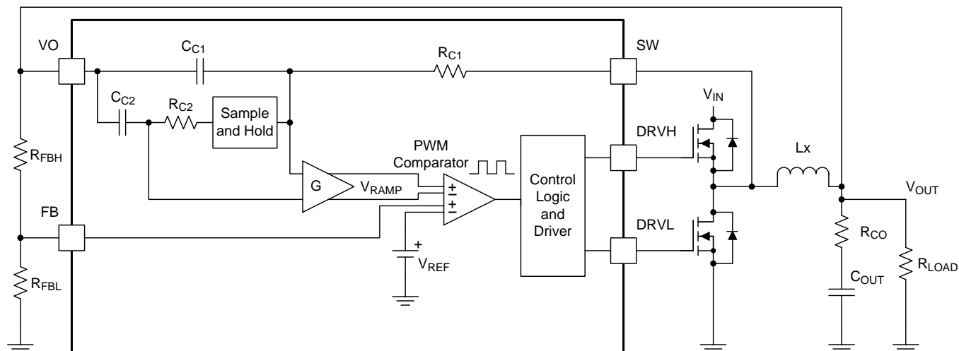
图 32. D-CAP3 Mode
