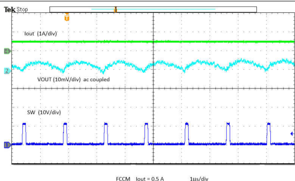
图 8-23. Output Voltage Ripple
