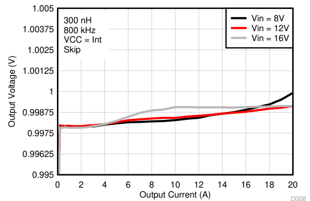
图 8-7. Output Voltage vs Output Current
