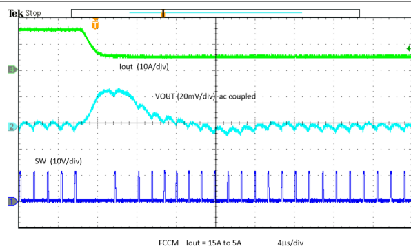
图 8-21. Unload Transient
