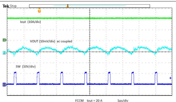
图 8-24. Output Voltage Ripple
