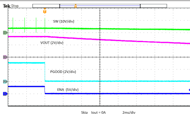
图 8-17. Enable Power Down, Skip
