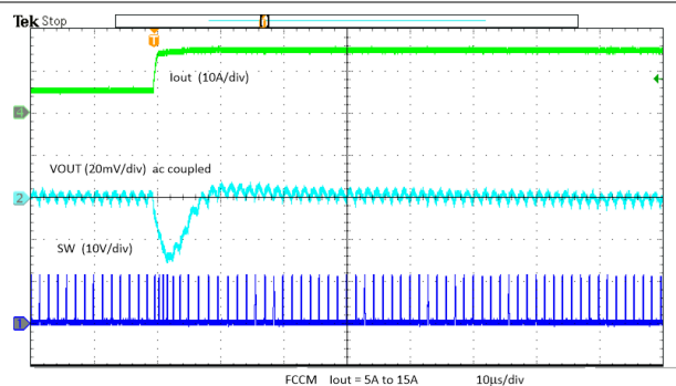
图 8-20. Load Transient
