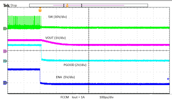
图 8-15. Prebias Power-Down
