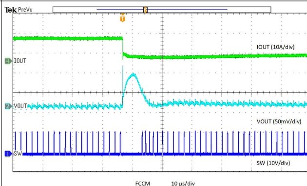
图 6-12. Unload Transient
