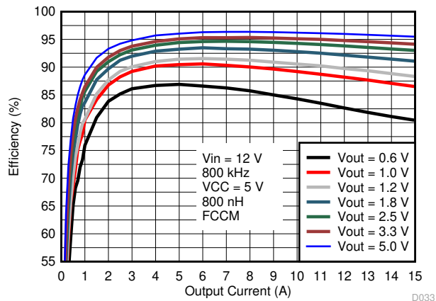
图 8-2. 效率与输出电流间的关系, V_{CC} = 5.0\text{V} 外部 VCC 偏置
