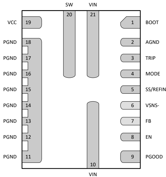
图 5-2. RWW 封装 21 引脚 VQFN-HR 底视图
