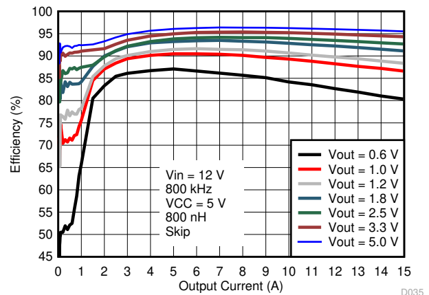
图 8-3. 效率与输出电流间的关系, V_{CC} = 5.0\text{V} 外部 VCC 偏置
