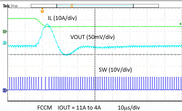
图 8-25. 空载瞬态
