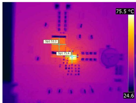
图 10-2. 25°C 环境温度下的热图像
