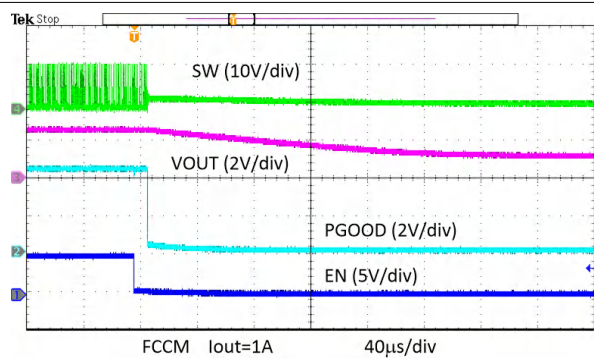
图 8-19. 预偏置上电
