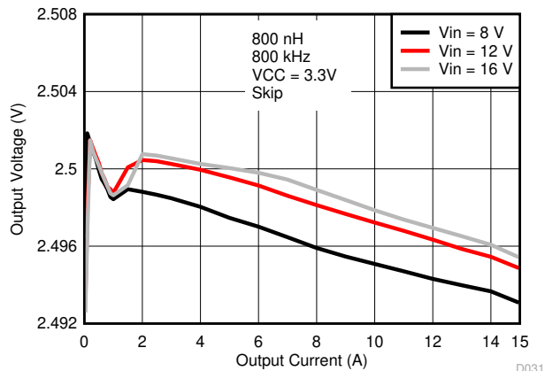
图 8-9. 输出电压与输出电流间的关系, VCC = 3.3V 外部偏置
