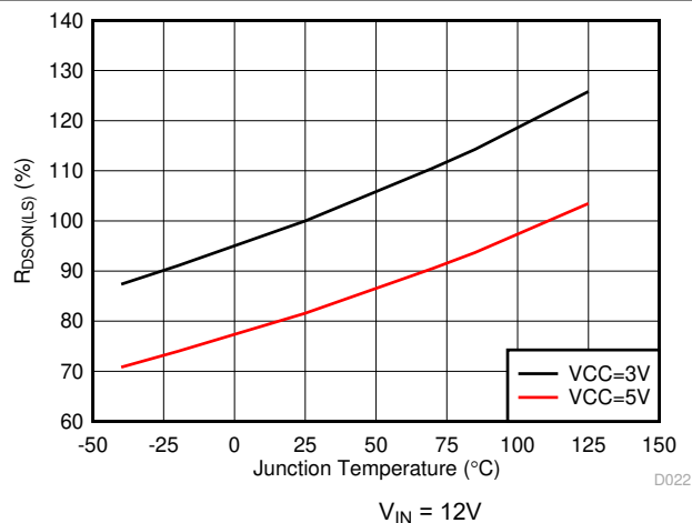
图 6-14. R_{DS(on)(LS)} 与结温间的关系
