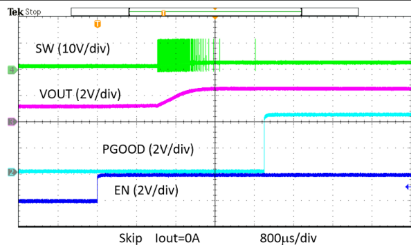
图 8-22. 使能上电至预偏置，跳越
