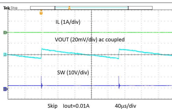
图 8-29. 输出电压纹波, 跳跃
