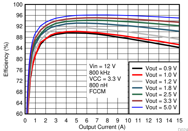
图 8-2. 效率与输出电流间的关系, V_{CC} = 3.3\text{ V} 外部 VCC 偏置
