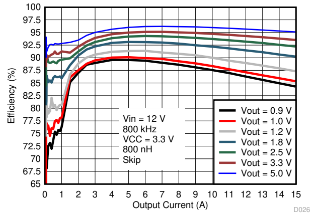
图 8-3. 效率与输出电流间的关系, V_{CC} = 5.0\text{ V} 外部 VCC 偏置
