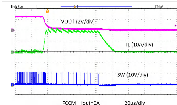
图 8-32. 过流保护
