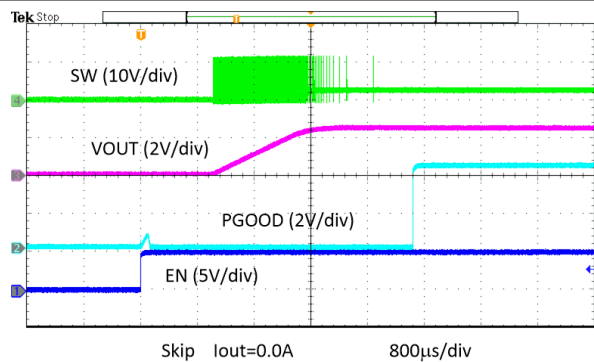
图 8-20. 使能上电，跳越
