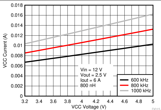
图 8-13. ICC 电流与外部 VCC 电压间的关系
