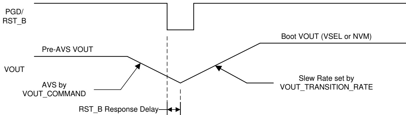
图 7-7. TPS546D24S Output Voltage Reset
