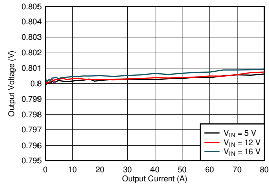
图 8-13. Load Regulation
