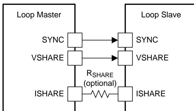
图 30. Current Sharing
