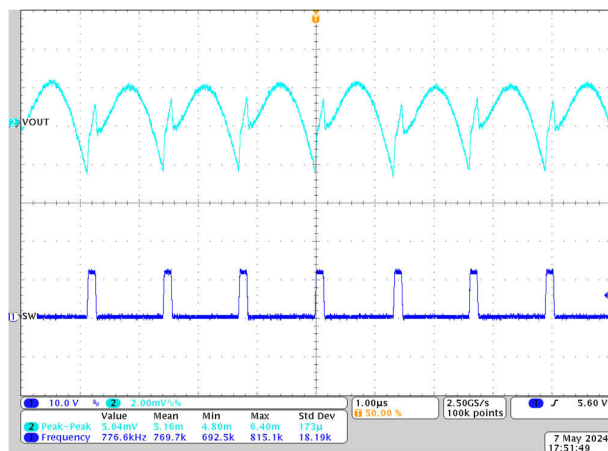
图 8-6. 输出电压纹波，1.2V Vout，800kHz FCCM，25A 负载
