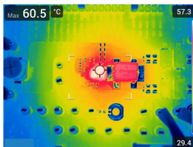
图 8-9. 热特性，800kHz FCCM，内部 LDO，25A 负载
