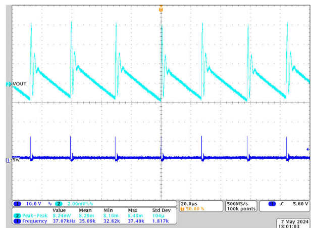
图 8-7. 输出电压纹波，1.2V Vout，800kHz DCM，空载
