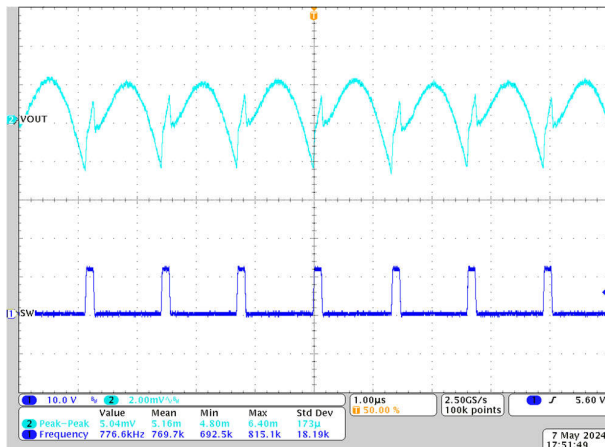
图 8-3. 输出电压纹波，1.2V Vout，800kHz FCCM，25A 负载
