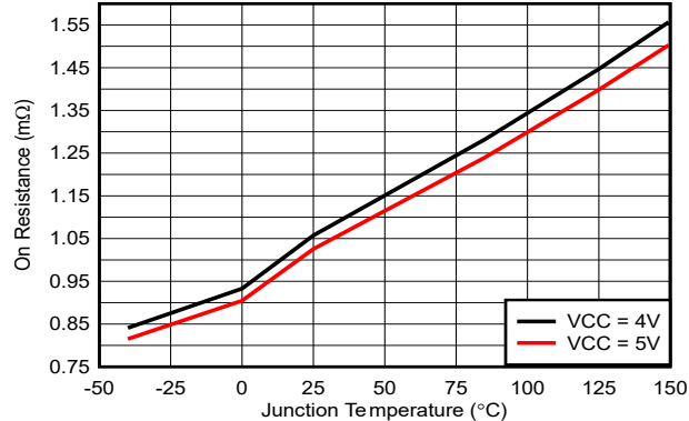
图 5-1. 低侧 MOSFET 导通电阻 ( R_{DS(on)} ) 与结温间的关系
