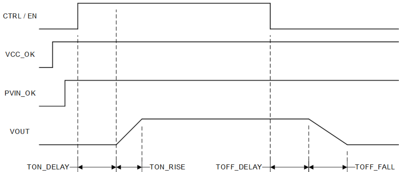
图 6-4. TPS546B25W 启动和关断
