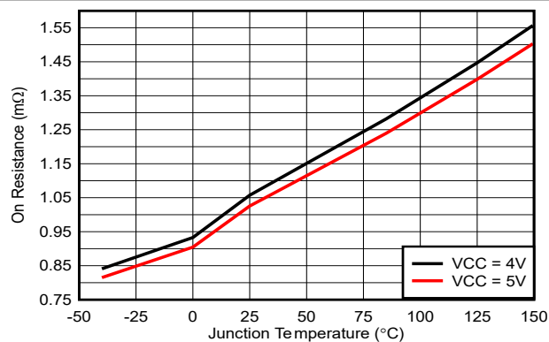
图 5-1. 低侧 MOSFET 导通电阻 ( R_{DS(on)} ) 与结温间的关系
