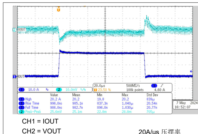
图 8-2. 负载瞬态，0A 至 20A
