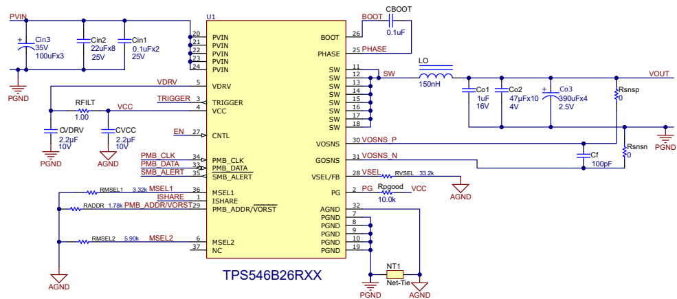
图 8-1. 1.2V、25A 输出应用
