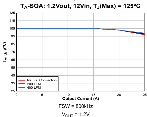
图 5-3. 安全工作区环境温度与负载电流间的关系
