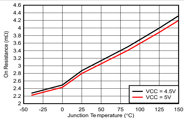
图 5-2. 高侧 MOSFET 导通电阻 ( R_{DS(on)} ) 与结温间的关系
