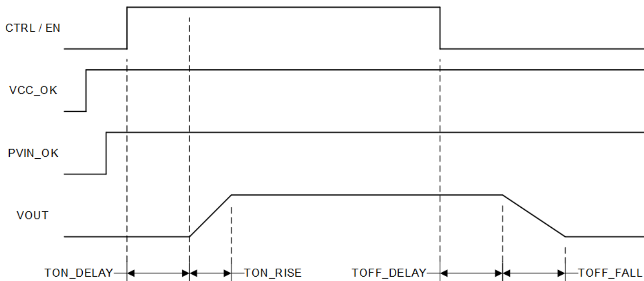
图 6-4. TPS546B25 启动和关断
