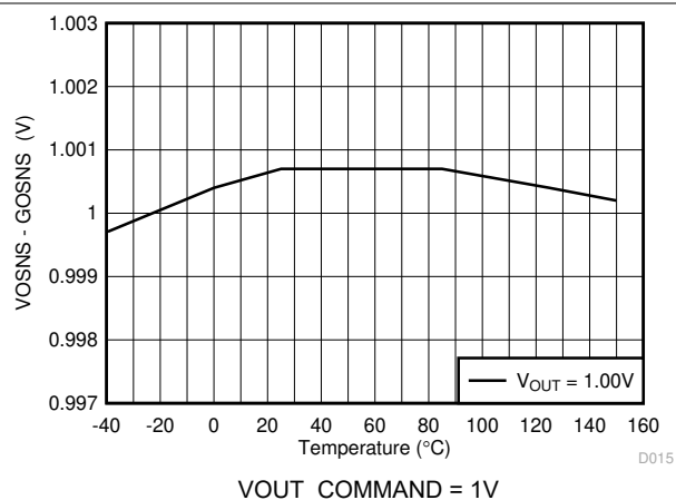
图 5-8. 输出电压与结温间的关系
