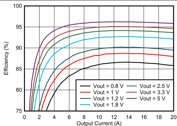
图 6-4. TPS546B24A 效率与输出电流间的关系
