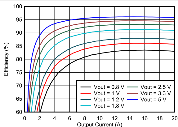
图 6-5. TPS546B24A 效率与输出电流间的关系
