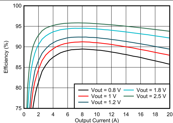
图 6-3. TPS546B24A 效率与输出电流间的关系
