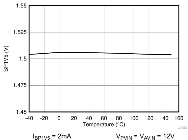
图 6-12. BP1V5 电压与结温间的关系
