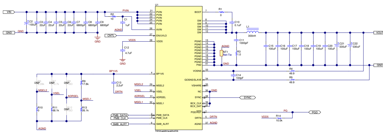
图 8-1. TPS546B24A 应用
