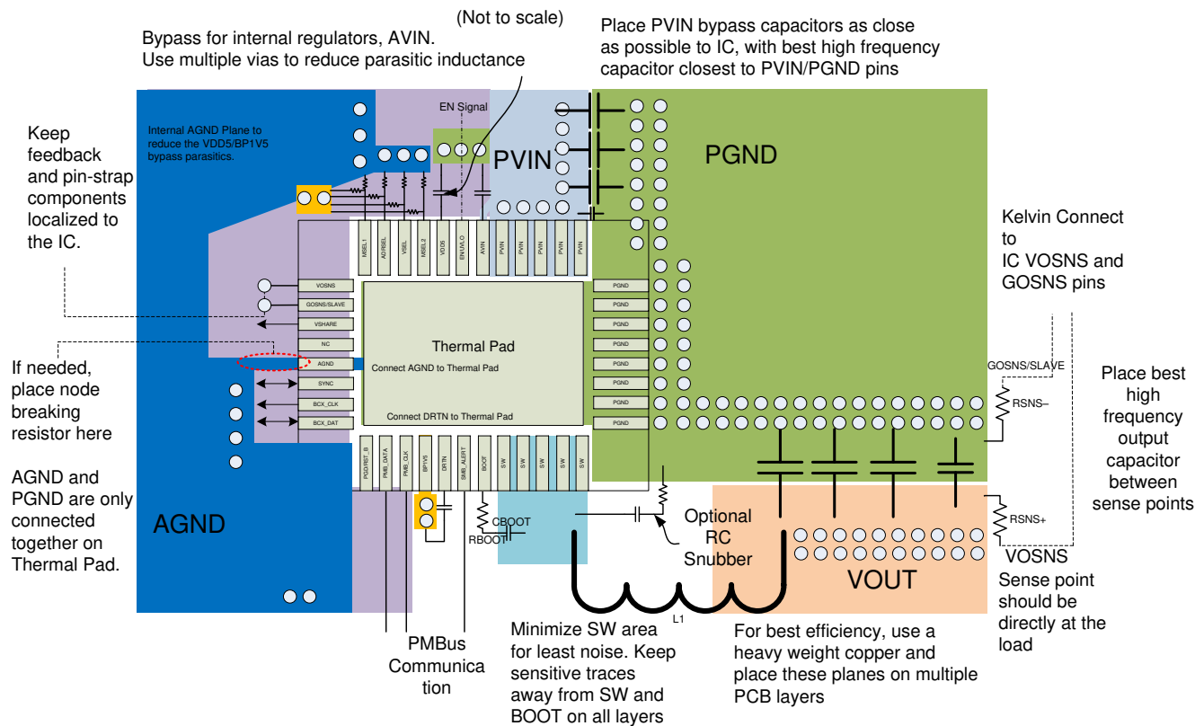
图 10-1. PCB 布局建议
