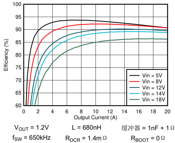
图 8-2. 效率与输出电流间的关系
