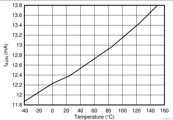
图 6-10. 非开关输入电流 ( I_{AVIN} ) 与结温间的关系
