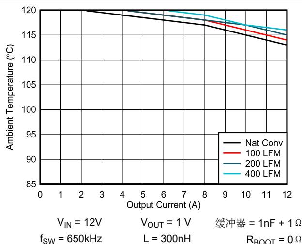
图 6-1. TPS546B24A 安全工作区
