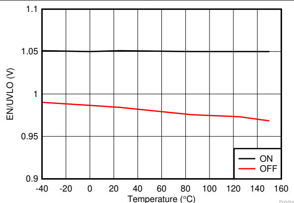
图 5-15. EN/UVLO 阈值与结温间的关系
