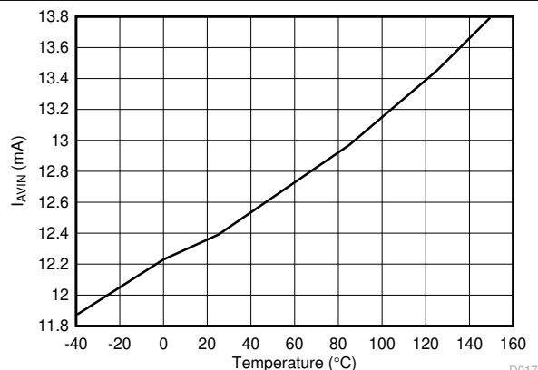
图 5-10. 非开关输入电流 ( I_{AVIN} ) 与结温间的关系
