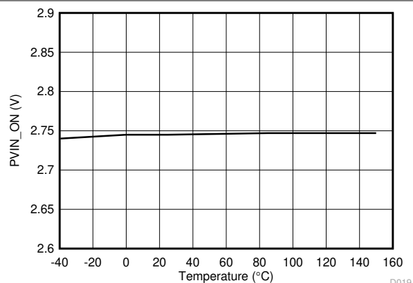
图 5-13. 导通电压与结温间的关系
