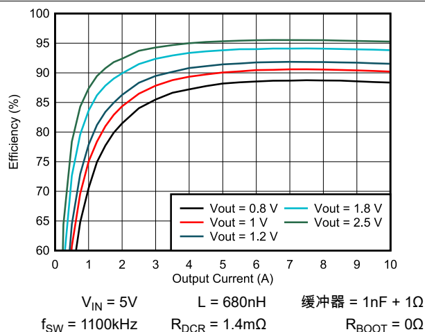
图 5-3. TPS546A24S 效率与输出电流间的关系
