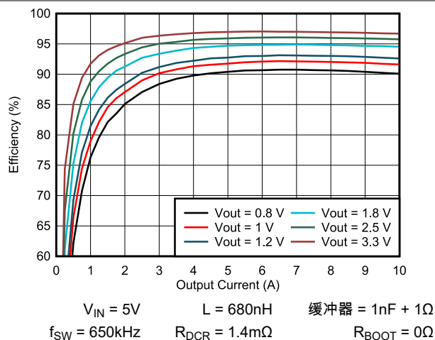
图 5-2. TPS546A24S 效率与输出电流间的关系
