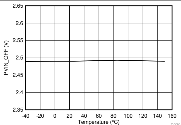
图 5-14. 关断电压与结温间的关系
