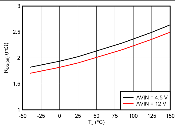
图 5-6. 低侧 MOSFET 导通电阻 ( R_{DS(on)} ) 与结温间的关系
