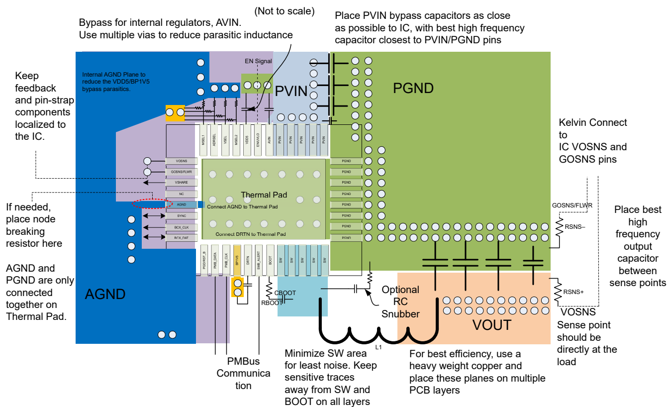
图 7-9. PCB 布局建议
