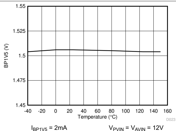
图 5-12. BP1V5 电压与结温间的关系
