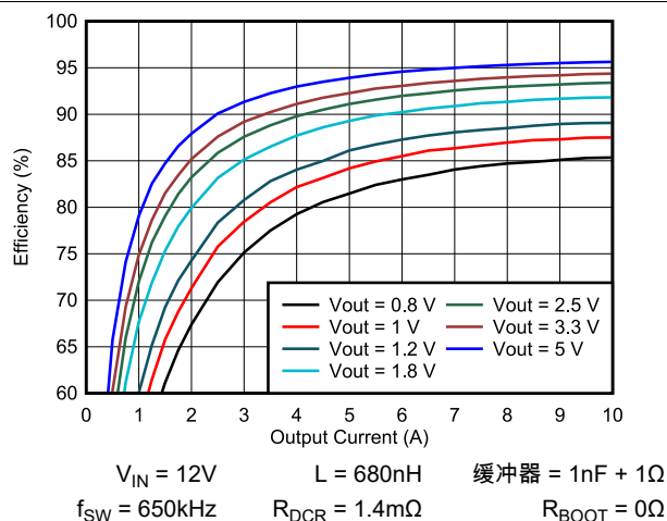
图 5-4. TPS546A24S 效率与输出电流间的关系
