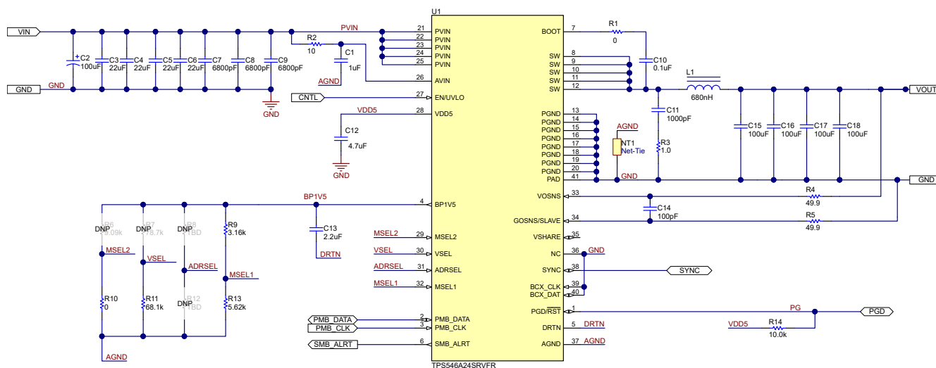
图 7-1. TPS546A24S 应用
