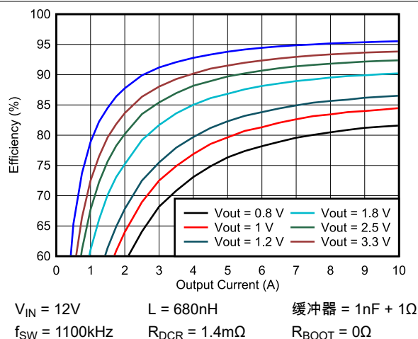
图 5-5. TPS546A24S 效率与输出电流间的关系
