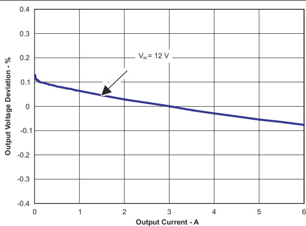
图 8-10. Load Regulation
