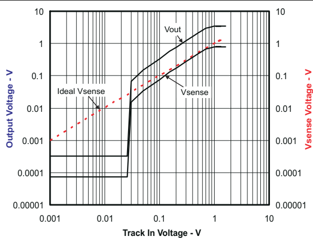
图 8-11. Tracking Performance
