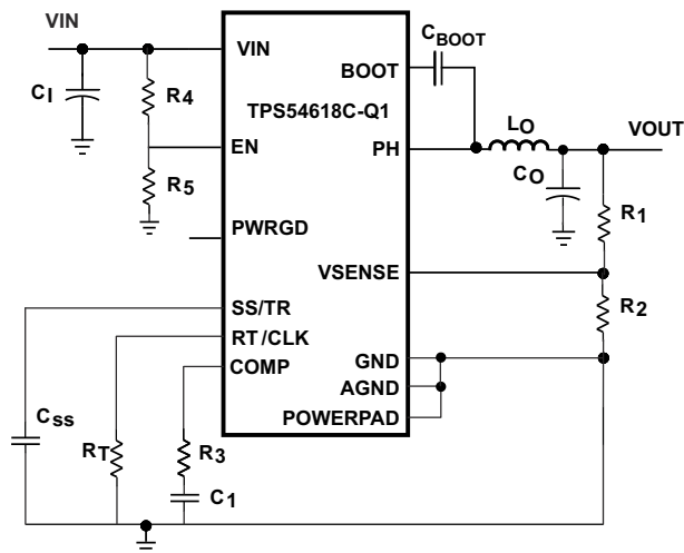
简化原理图
