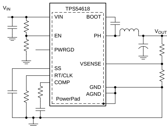
简化原理图
