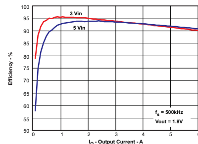
效率与输出电流间的关系
