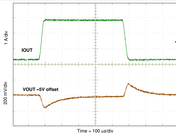
图 8-6. Load Transient
