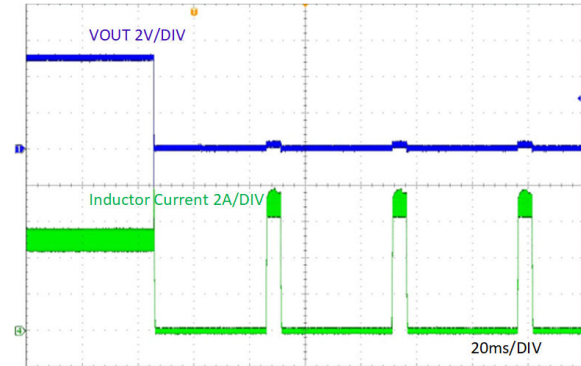
图 7-15. V OUT 硬短路保护
