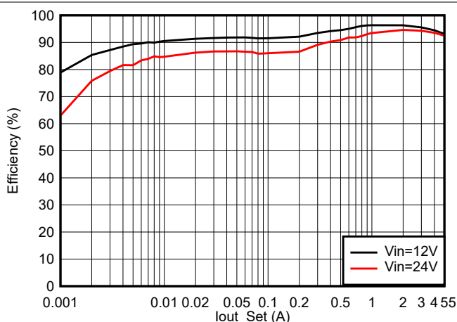
图 7-2. 效率 (PFM)
