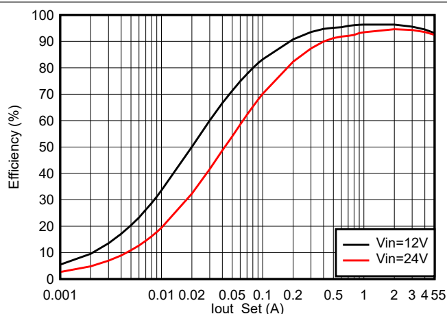
图 7-3. 效率 (FCCM)
