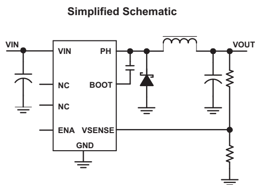
简化原理图和效率曲线
